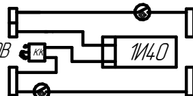
Рисунок 6. ЛПО46-2x18 (Применять по требованию заказчика)
