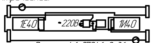
Рисунок 4.1 ЛПО46-2x36
