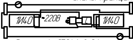
Рисунок 4. ЛПО46-2x36
