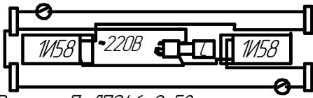
Рисунок 7. ЛПО46-2x58
