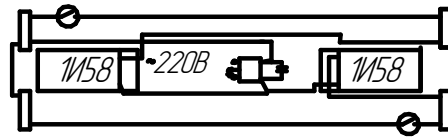
Рисунок 8. ЛПО46-2x58 (Применять по требованию заказчика)
