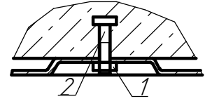
Рисунок 3. Крепление светильника на монтажную поверхность: 1.Гайка. 2.Болт.
