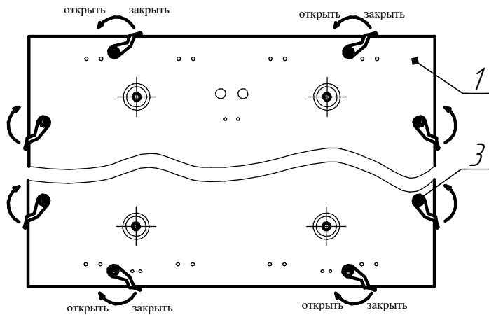
Рисунок 1. 2: ЛПО46-4x14; 1. Корпус в сборе; 3. Зажим
