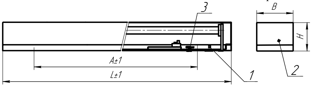
Рисунок 1. ЛПО46-1x54; 2x14; 2x28; 2x54
