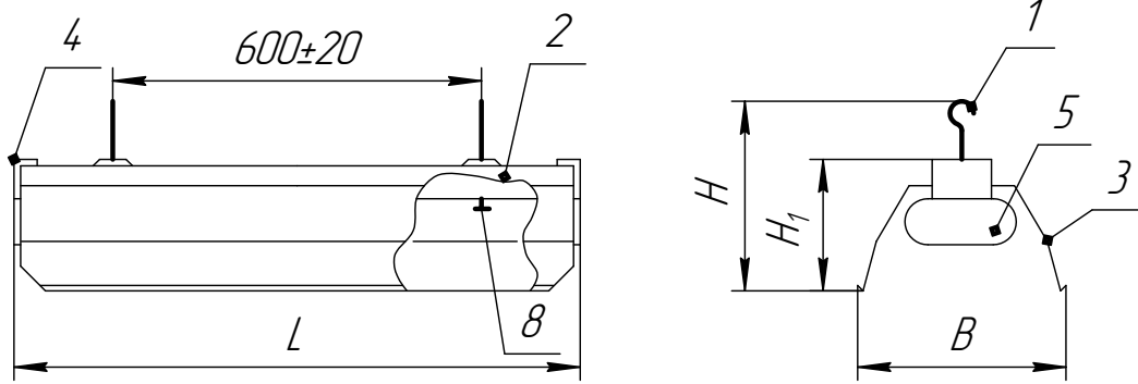
Рисунок 1: 1. Узел подвеса; 2. Корпус; 3. Отражатель; 4. Крышка торцевая; 5. Скоба с патронами; 8. Винт специальный.
