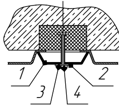
Рисунок 7 – Крепление светильника на горизонтальную поверхность: 1. Швеллер; 2. Шайба; 3. Гайка; 4. Болт.
