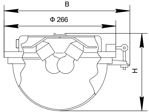
Рисунок 2. НПП03-2x40-001, НПП03-2x40-002.
