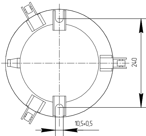
Рисунок 4. - установочные размеры.
