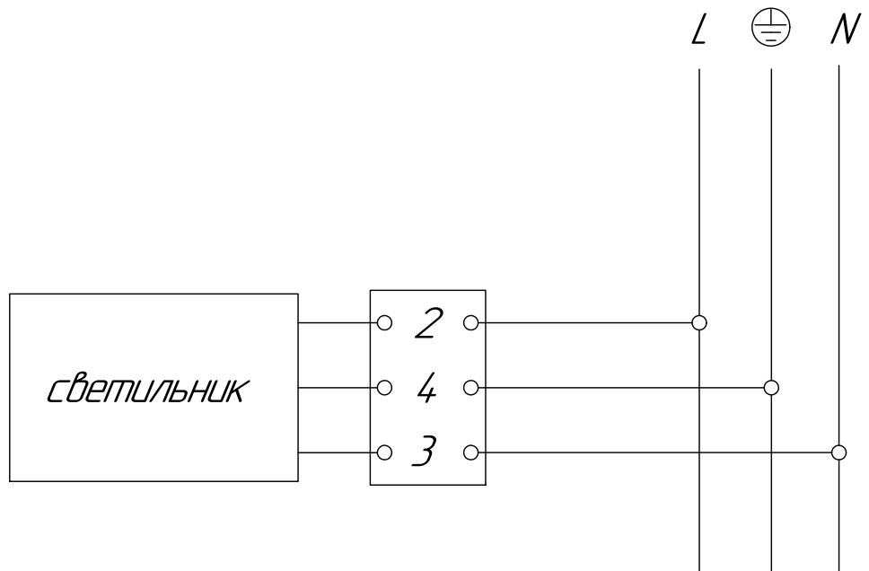
Рисунок 2 - Схема подключения прожектора к сети
