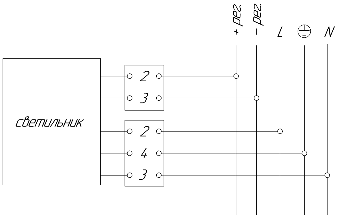
Рисунок 3 - Схема подключения прожектора с управлением к сети
