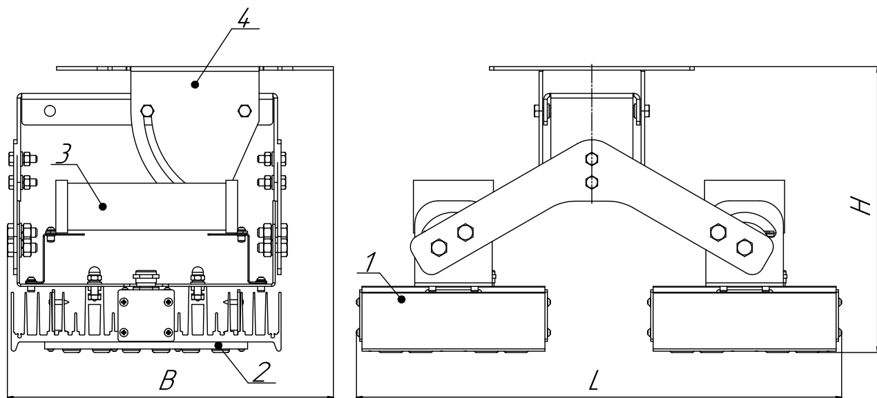
Рисунок 1в - Внешний вид и габариты прожекторов серии ДО15 мощностью 2x40, 2x80 Вт.
