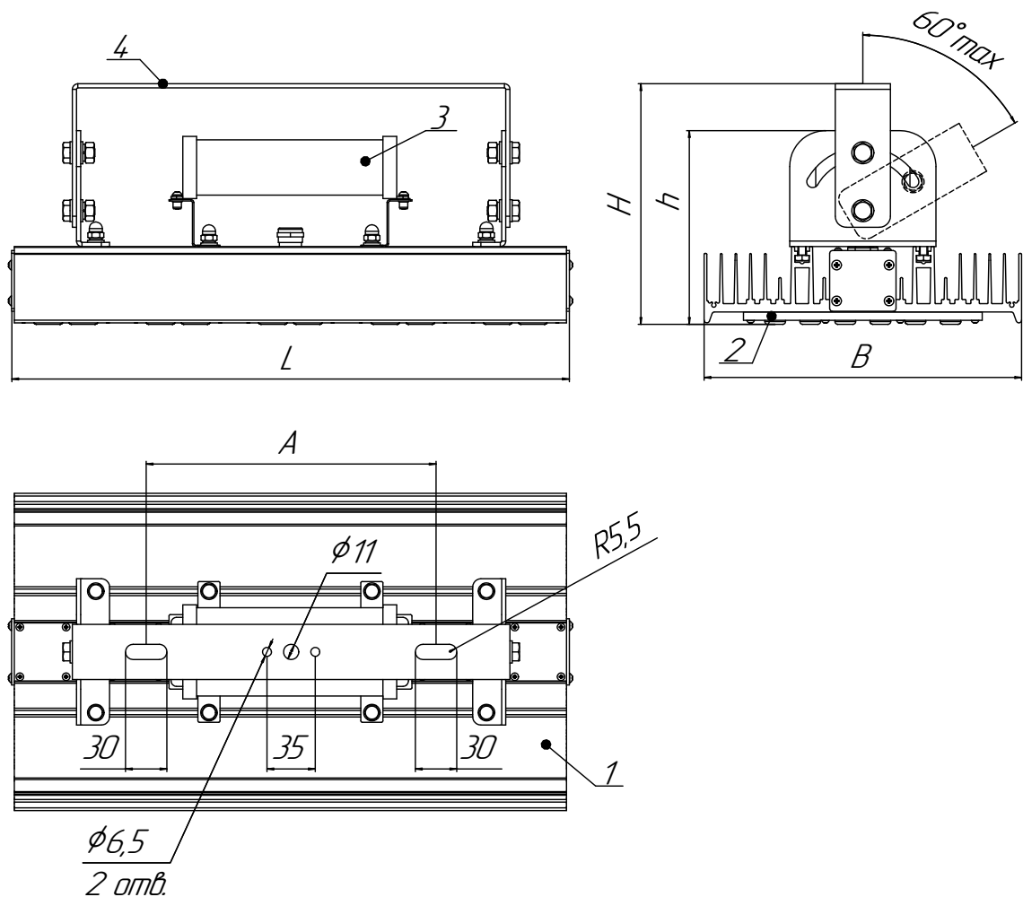
Рисунок 1б - Внешний вид и габариты прожекторов серии ДО15 мощностью 120, 160, 200, 240 Вт.
