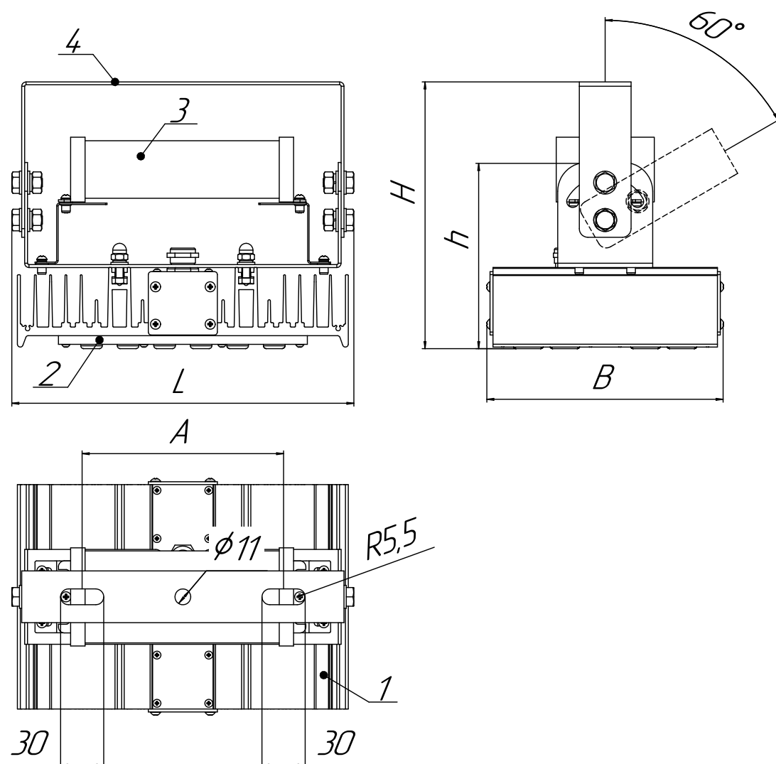
Рисунок 1а - Внешний вид и габариты прожекторов серии ДО15 мощностью 40, 80 Вт.
